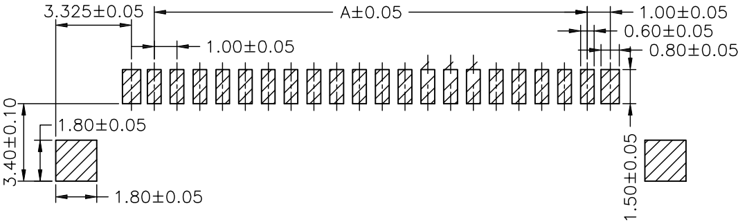
P.C.B LAYOUT
